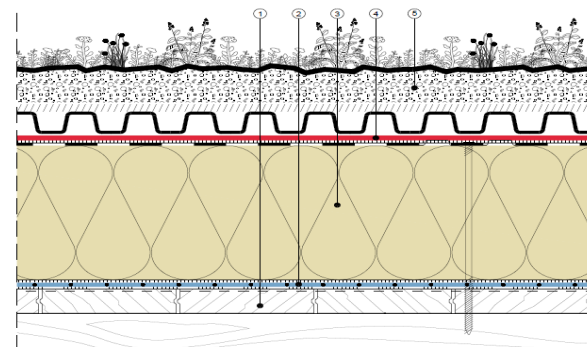
Масштаб 1:2.5 (Размер гидроизоляции EPDM представлен преувеличенным)
