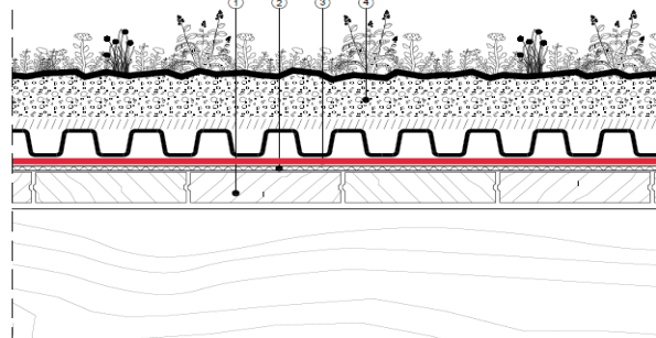
Масштаб 1:2.5 (Гидроизоляционная мембрана EPDM преувеличена в размерах)
